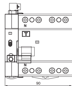
EKR5 + EKL6-100 4P EKR5 + EKL6-100B 4P EKR5 + EKL6-63EV 4P
